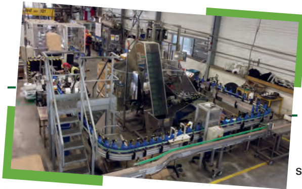
Usine de Bourth (27) Production d'engrais, de produits de soin des plantes et d'anti-nuisibles
